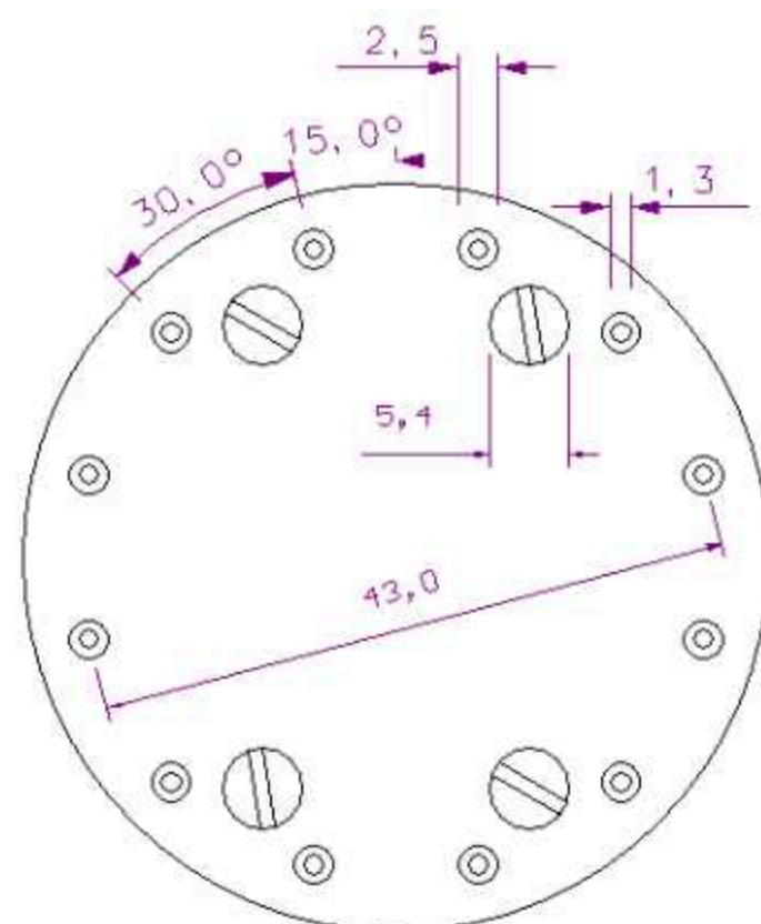
Foratura consigliata PCB 1,7mm
