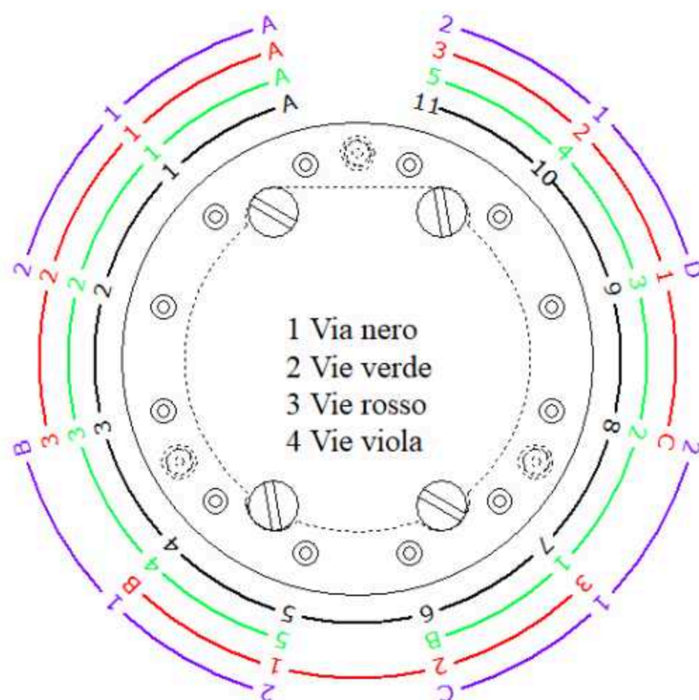
Connessioni viste lato saldature
